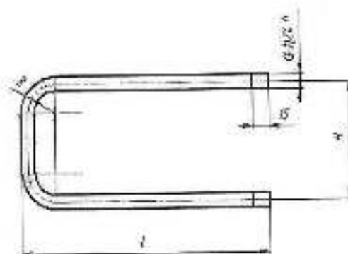
Общий вид П-обр.
